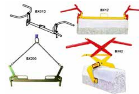
Pinces BX (EN 13155) Pour la manutention et la pose de bordures. Taille normalisée de longueur 1 m. Avec au choix : poignées, guidons ou système utilisable avec jeu de levage en chaîne qui facilitent la manutention.
