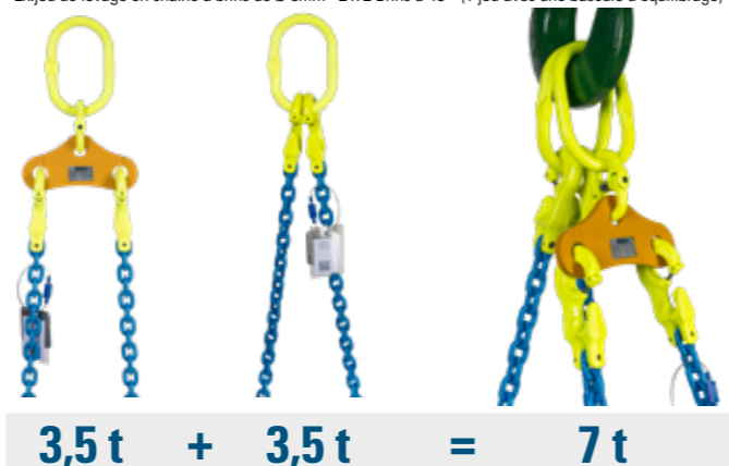
Ex. jeu de levage en chaîne à brins de Ø 8mm - 2 x 2 Brins à 45° (1 jeu avec une bascule d'équilibrage)
