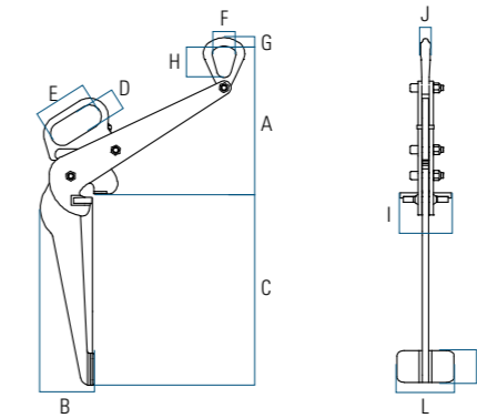
Pince VLF pour le levage de fûts (EN 13155) Pour fûts en acier à rebord, de diamètre 600 mm, pleins ou vides - en position verticale. Utilisation en batterie avec palonnier possible. Elle est équipée d'un système de pincement du rebord du fût. Une poignée permet la mise en place sur le fût et le déverrouillage de la pince sur celui-ci. Le serrage de la pince est proportionnel à la charge limitant ainsi le risque de dommage.
