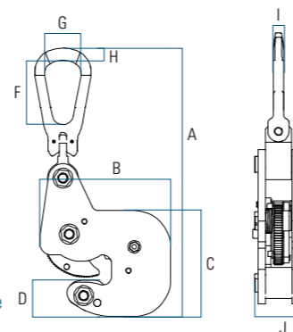
Pince semi-automatique pour levage de profilés (EN 13155) Levage de profilés en I ou H ou d'ensembles mécano-soudés, de tôles en position horizontale. Avec système de sécurité par ressort permettant un contact permanent de la came sur la pièce à lever, même lors de la dépose de celle-ci. Avec système de prise automatique assurant la fermeture de la pince lorsque le profilé ou la tôle sont positionnés en fond de gorge. Peut être utilisée à un angle de min 30° à max 45°.
