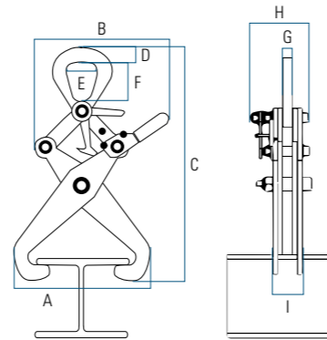
Pince PL semi-automatique pour poutrelle (EN 13155) Pour profil H et I. Avec système de verrouillage très pratique qui permet de déposer la charge sans intervention. Avec poignée pour faciliter la mise en place. Employer par paire (palonnier conseillé).
