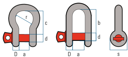
Fig. 4: Droite, avec boulon et goupille
