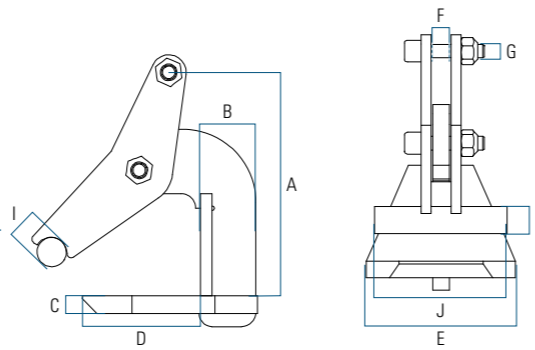
Pince à tôle TLH (EN 13155) Pince pour levage de plaques horizontales. Prise réglable. Employer par paire. Peut être utilisée à un angle de minimum 22,5° à 30°. Sur demande avec prise de 0 - 120 mm et 0 - 150 mm
