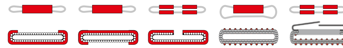
Fourreau SF-1, avec protection secutex® 1 face, protège contre les arêtes vives. Fourreau SF-2, avec protection secutex® 2 faces, protège contre les arêtes vives. Fourreau SC Clip avec protection secutex® 1 face, fendu sur un côté pour montage facile. Protège contre les arêtes vives. Fourreau NoCut® sleeve 2 faces. Flexible, léger. La meilleure protection contre les charges tranchantes. Protection NoCut® pad est appliquée exactement à l'endroit nécessaire
