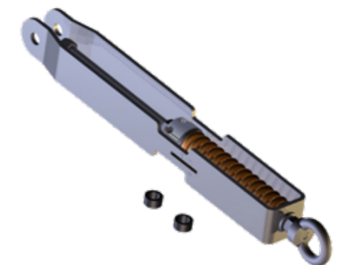
Coulisseau amovible
