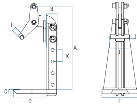
Pince TLR (EN 13155) Pince pour levage de plaques horizontales. Prise réglable. S'utilise par paire. Peut être utilisée à un angle de minimum 22,5° à 30°.
