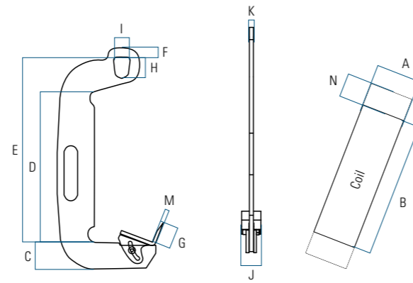
Clé de retournement CR (EN 13155) Pour levage et retournement de coils. Avec bec de sécurité et une poignée de positionnement pratique.
