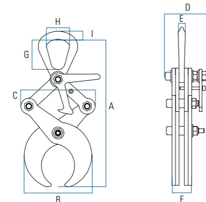
Pince pour matériaux rond RT (EN 13155) Pour levage de tuyaux et pose en tranchées. La pince s'ouvre automatiquement dès que la charge est déposée. Livrable sur demande avec une capacité de 3000 kg. Employer par paire (palonnier conseillé)
