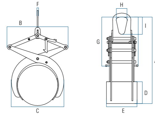
Pince pour tuyau TI (EN 13155) Pour levage de tuyaux et pose en tranchées. Disponible en variante semi ou complètement automatique TIS = semi-automatique TIA = automatique
