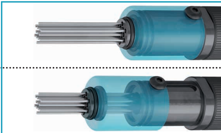
Le coulisseau à aiguille réglable avec guidage d'aiguille intégré garantit de longues durées de vie
