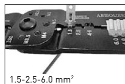
Quetschzange für nicht isolierte Kabelschuhe Sertissage pour cosse nues Pinza a crimpare per terminali a barre
