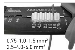
Abisolierzange für Kabel Dénudage de câbles Spelafili per cavi
